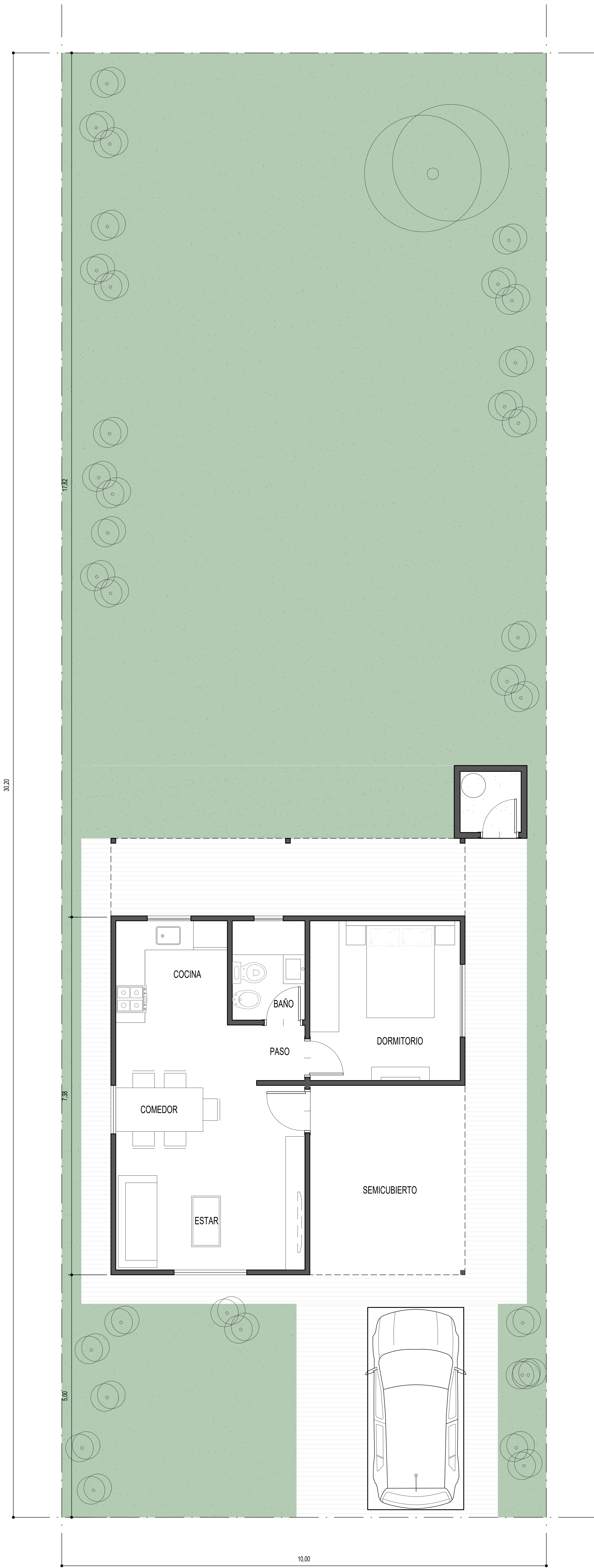
IMPLANTACION PROYECTO 40M2
