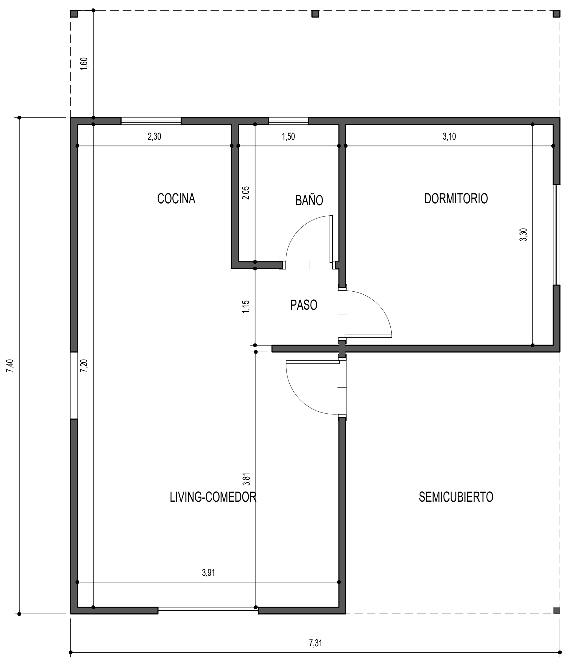
PLANTA ACOTADA
